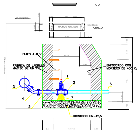
SECCION
