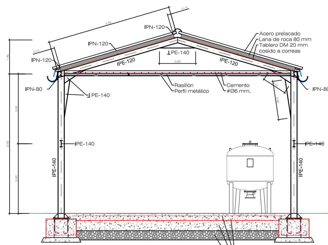
ESTRUCTURA PÓRTICO INTERIOR Escala= 1/50
