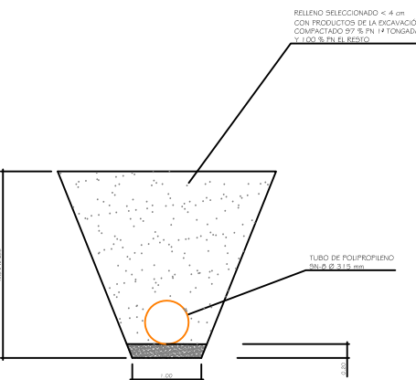
TALUDES
