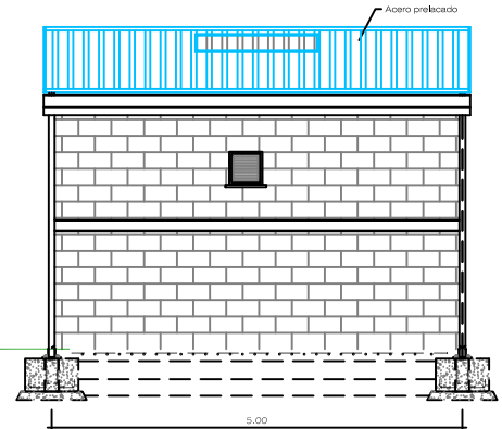
ALZADO LATERAL IZQUIERDO Escala= 1/100
