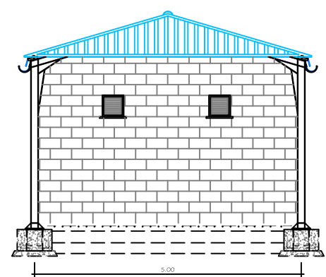
ALZADO POSTERIOR Escala= 1/100
