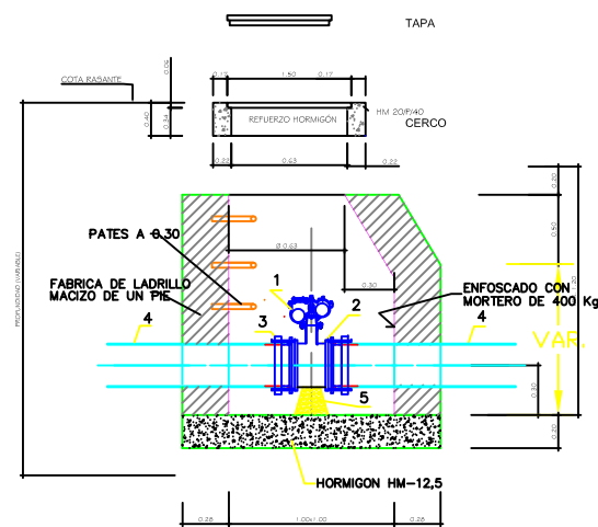
SECCION
